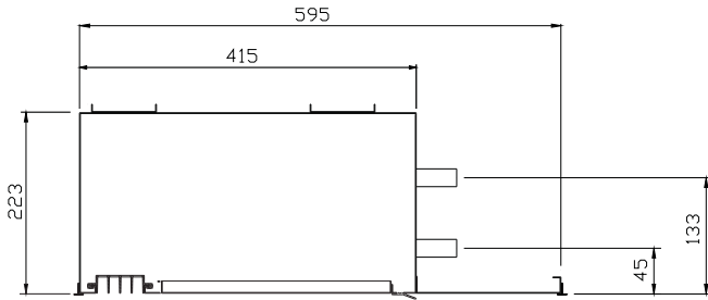
T-Bar: Void Inlet - Side Profile
